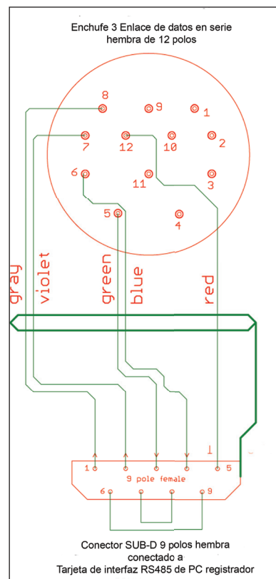
Fig. 11.4 Paso 3 Conexión de clavijas
